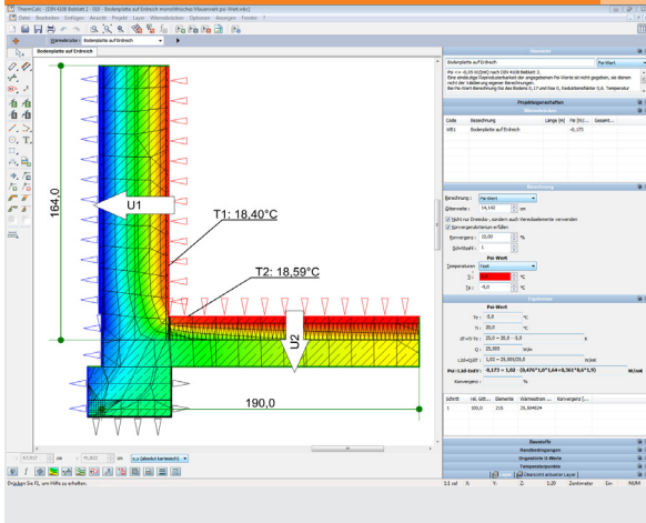
Dialog zum Berechnen einer 2D-Wärmebrücke (Bodenplatte gegen Erdreich). Darstellung der Wärmebrücke mit Isothermen, FEM-Gitter und Temperaturen an ausgewählten Oberflächen-Punkten.
